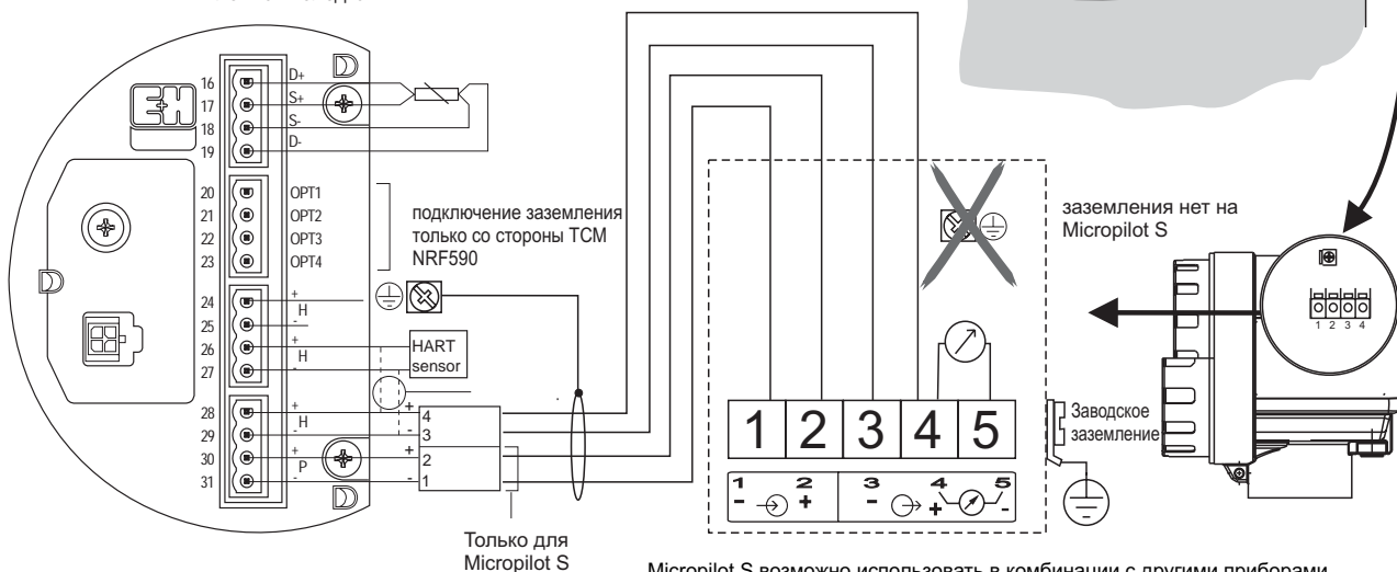
Искробезопасная клеммная колодка
