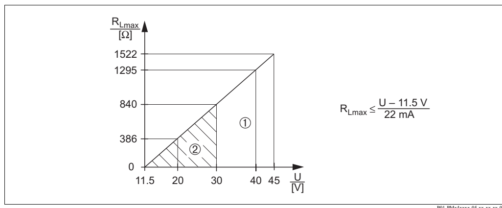
Нагрузочная диаграмма
