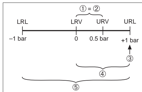
Пример: измерительная ячейка 1 бар
