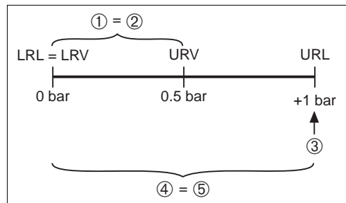
Пример: измерительная ячейка 1 бар
