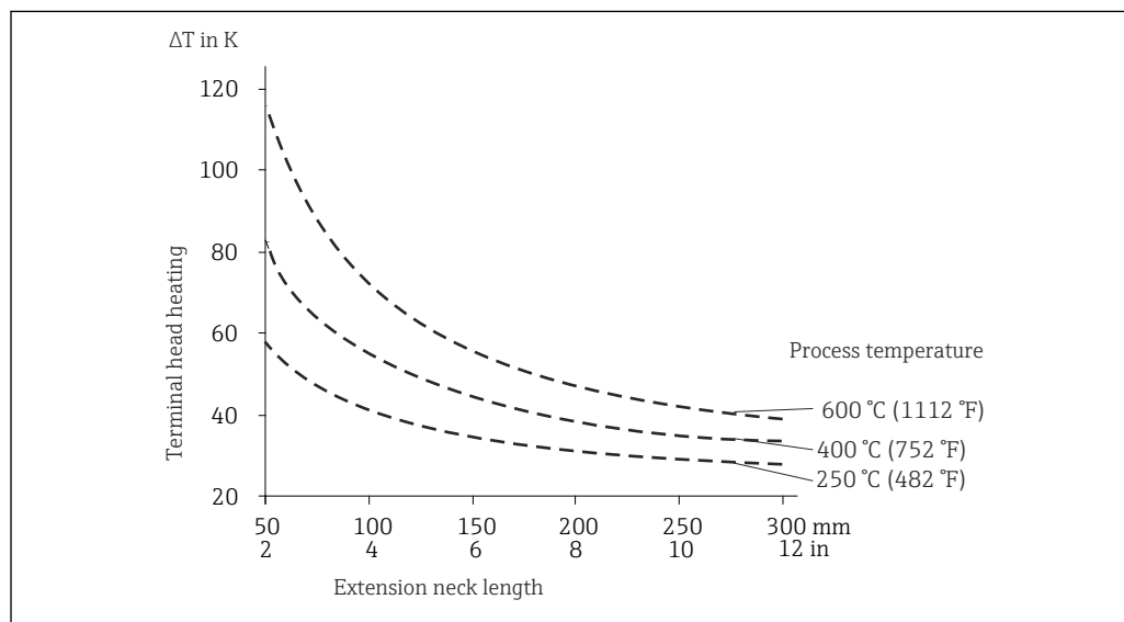
6 Нагрев присоединительной головки под воздействием рабочей температуры. Температура в клемной головке = температура окружающей среды 20 °C (68 °F) + ΔT
