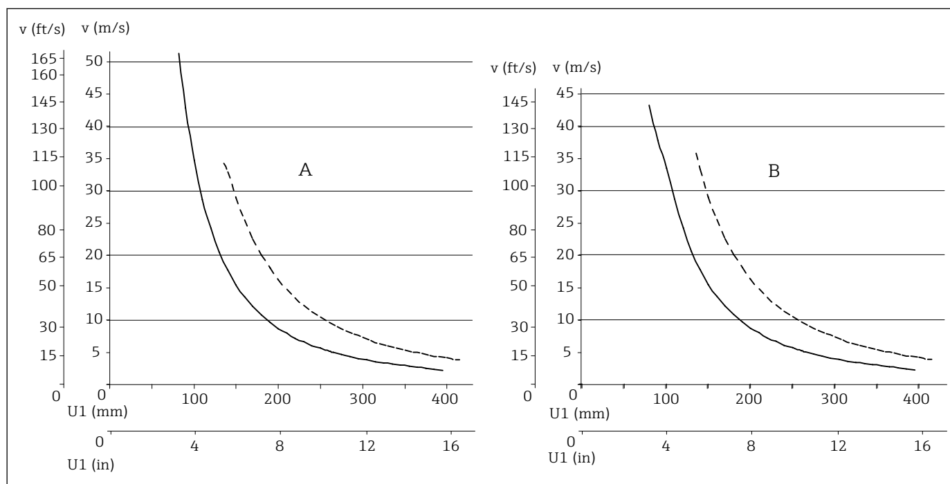
3 Допустимая скорость потока в зависимости от глубины погружения
