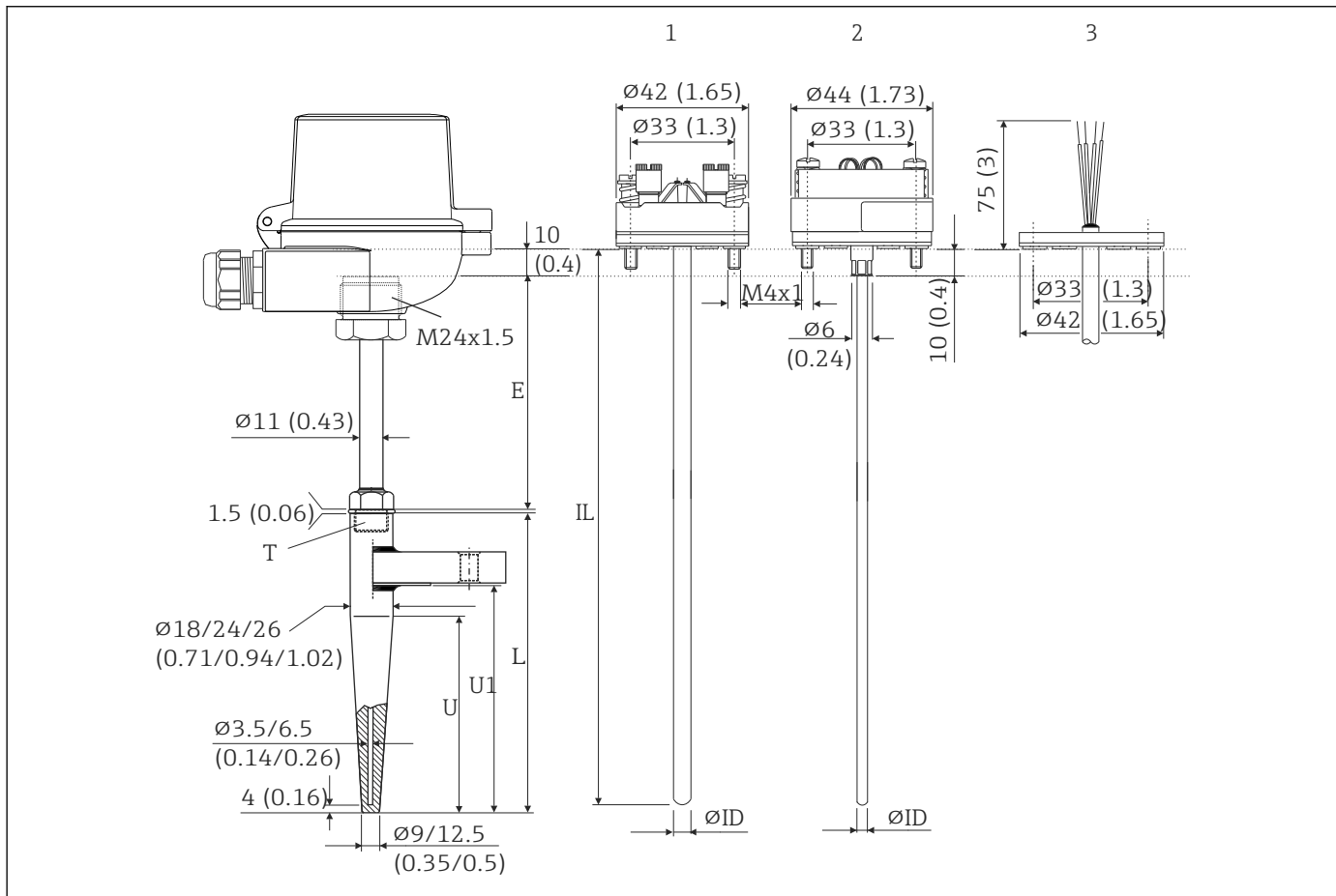
4 Размеры приборов Omnigrad M TR15 и TC15
