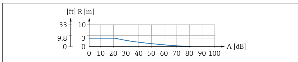
2 График диапазонов для ультразвуковых датчиков
