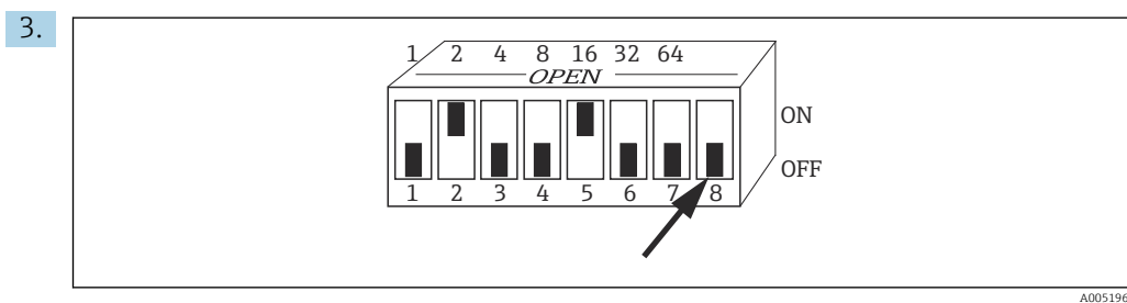
9 Пример настройки адреса прибора с помощью DIP-переключателя
