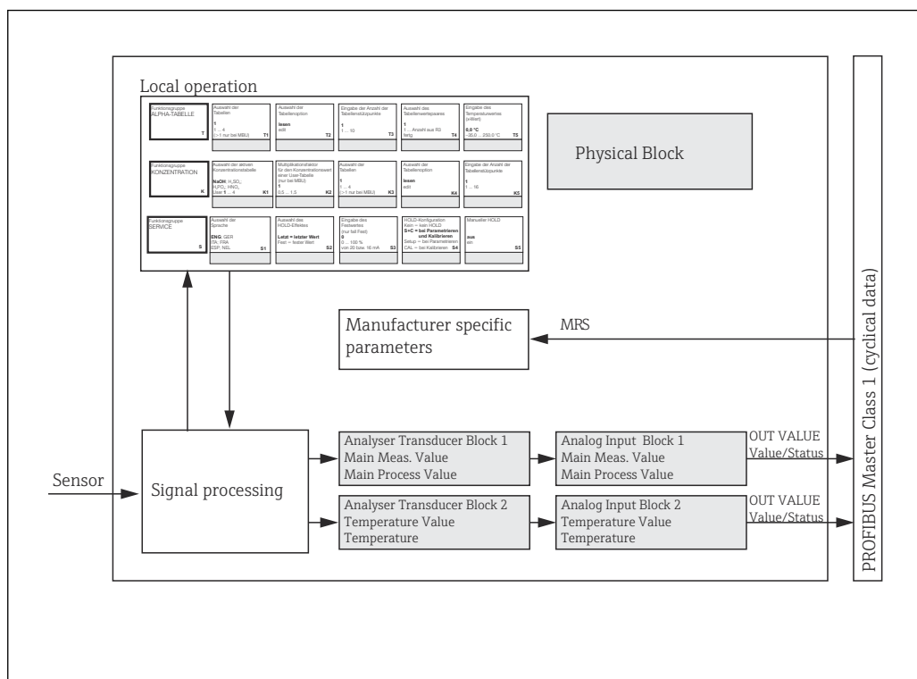
4 Блочная модель (серый – профильные блоки)
