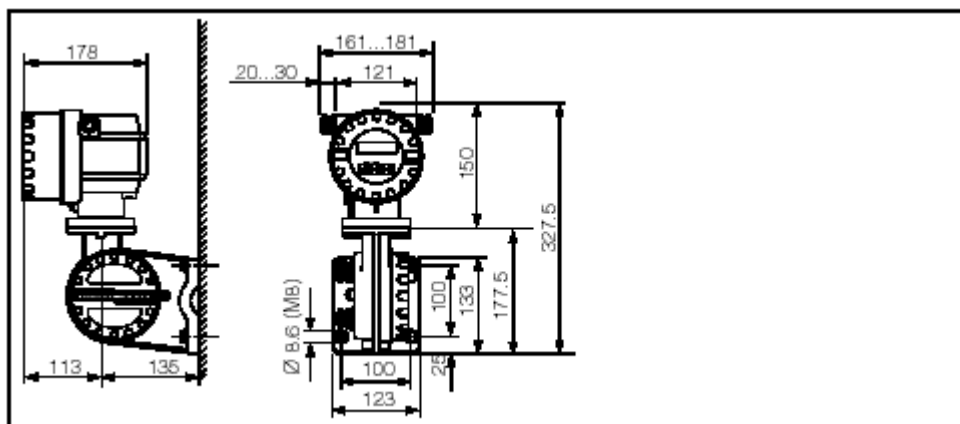
Размеры Promag 10 (раздельное исполнение)
