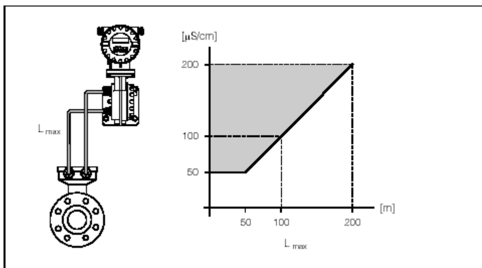
Допустимый диапазон для проводимости среды Площадь, окрашенная серым = допустимый диапазон L_{\text{max}} = длина соединительного кабеля в [м] Проводимость среды в [мкСм/см]
