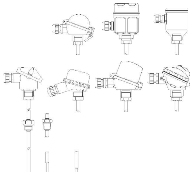
Рис. 1: TC 10 с различными типами головок, присоединений к процессу и кончиков термогильзы.
